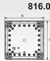
Gehäuse / Enclosure
